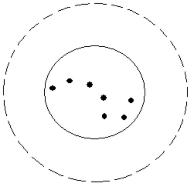
Orsa Maggiore
