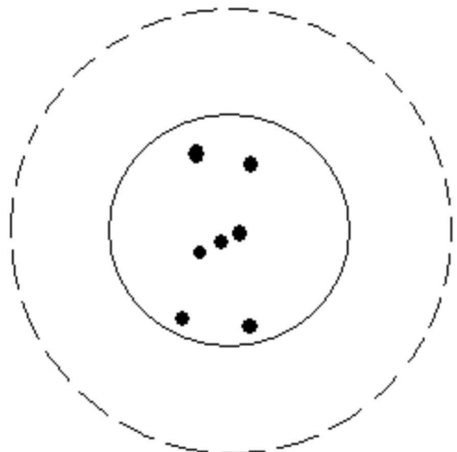
Orione
