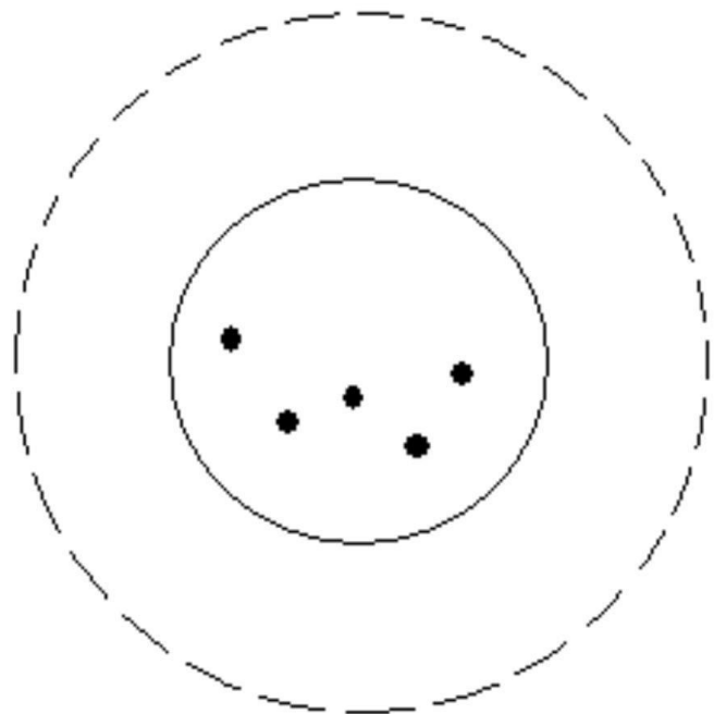
Cassiopea
